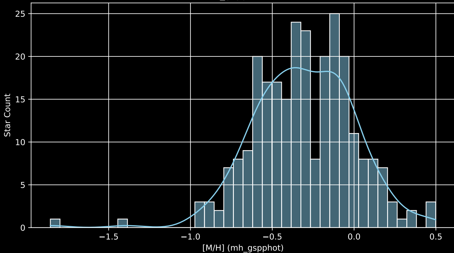
GALAH DR4 Field: [750] [M/H] (mh_gspphot) (n= 266)
