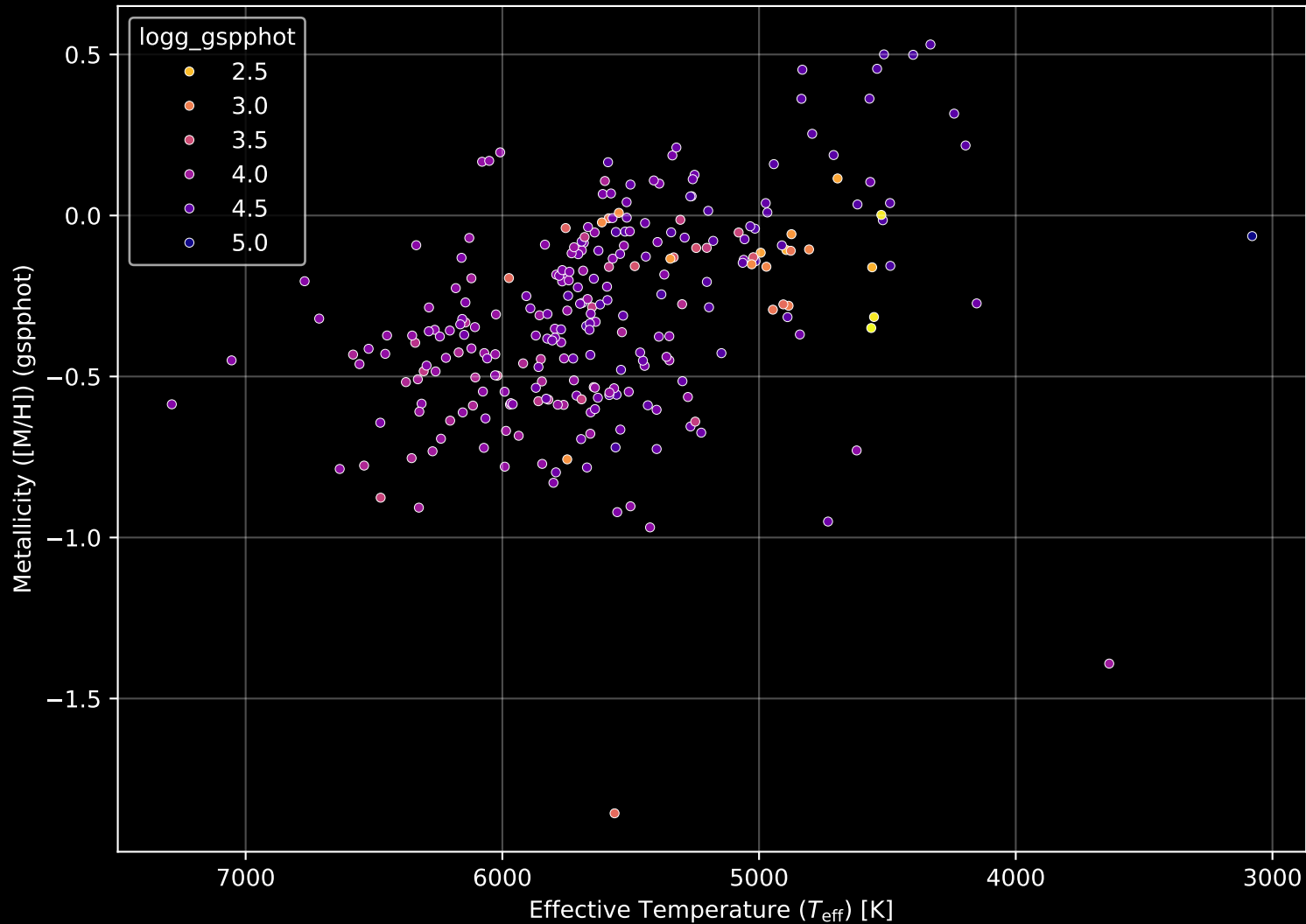
GALAH DR4 Field: [750] Stellar Population Parameters (n= 268)
