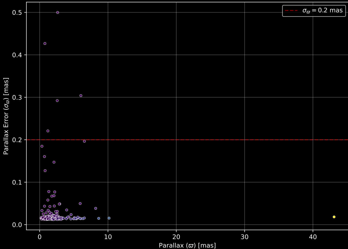
GALAH DR4 Field: [750] Parallax Quality (n= 268)
